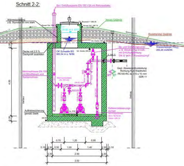
Schnitt 2-2:
